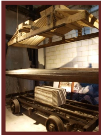
Armure à scier exposée au musée
